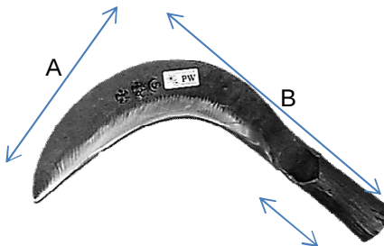
Sabit Rumput (tajam) Besi Spring 草镰刀 (尖咀)
