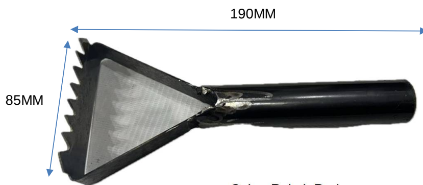
Cakar Pokok Durian 去寄生植物耙
